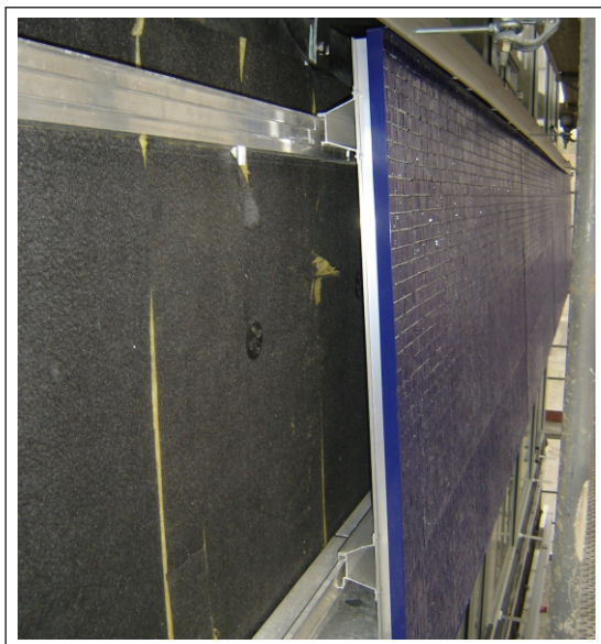
Brüstungsquerschnitt geneigte Elemente
