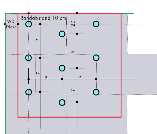
Dübelanzahl: 9 Stück/m 2 Dübelachsen: x = 33 cm; y = 33 cm
