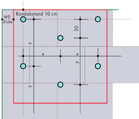
Dübelanzahl: 6 Stück/m 2 Dübelachsen: x = 40 cm; y = 50 cm
