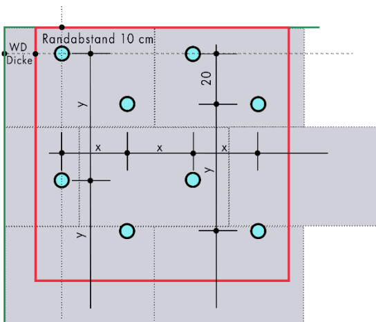
Dübelanzahl: 8 Stück/m 2 Dübelachsen: x = 26 cm; y = 50 cm
