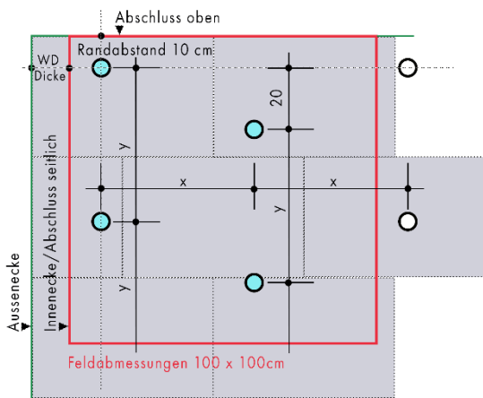
Dübelanzahl: 4 Stück/m 2 Dübelachsen: x = 50 cm; y = 50 cm
