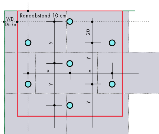
Dübelanzahl: 7 Stück/m 2 Dübelachsen: x = 40 cm; y = 40 cm
