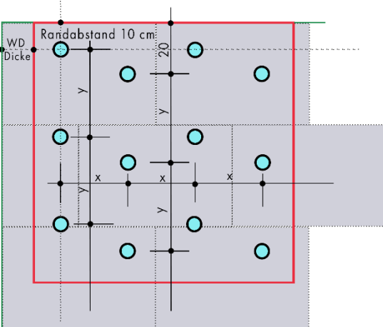
Dübelanzahl: 12 Stück/m 2 Dübelachsen: x = 26 cm; y = 34 cm
