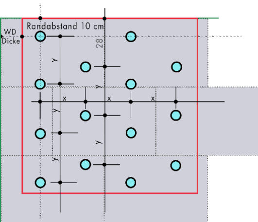
Dübelanzahl: 14 Stück/m 2 Dübelachsen: x = 26 cm; y = 28 cm
