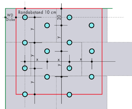
Dübelanzahl: 13 Stück/m 2 Dübelachsen: x = 26 cm; y = 30 cm
