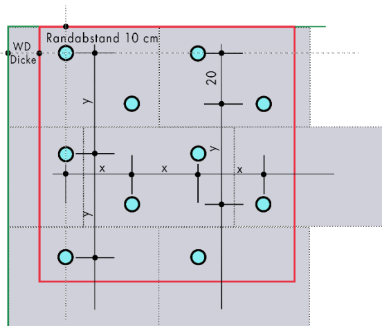
Dübelanzahl: 10 Stück/m 2 Dübelachsen: x = 26 cm; y = 40 cm
