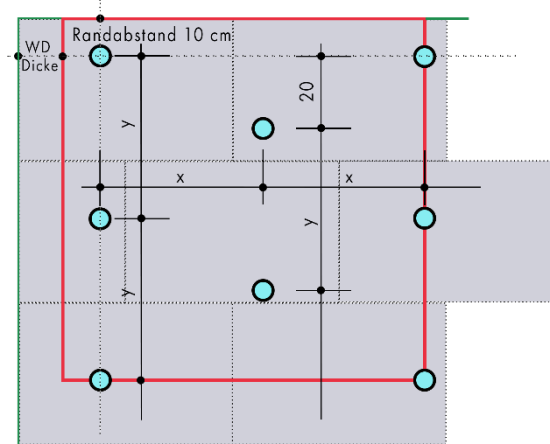
Dübelanzahl: 5.5 Stück/m 2 Dübelachsen: x = 45 cm; y = 45 cm
