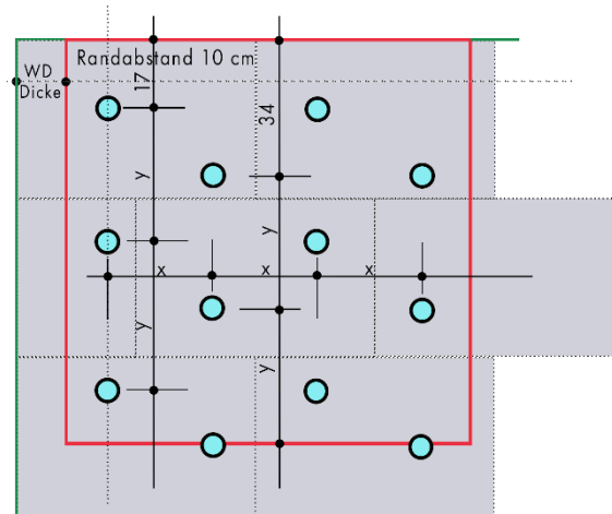
Dübelanzahl: 11 Stück/m 2 Dübelachsen: x = 26 cm; y = 33 cm
